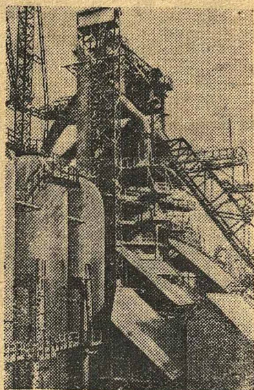
Румынская Народная Республика. Металлургический комбинат в Хунедоаре — одно из крупнейших предприятий страны. В этом году на комбинате введены в строй действующих новые производственные объекты, в том числе крупные доменные печи.
