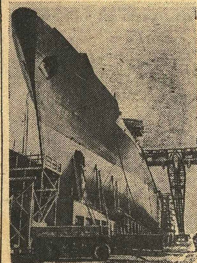
Германская Демократическая Республика. Недавно судостроительные верфи Росток спустили на воду грузовой корабль водоизмещением 10.000 тонн. Длина корабля 157,6 метра. Корабль имеет четыре дизельных мотора по 2.400 лошадиных сил каждый. Скорость корабля до 18,5 миль в час.
